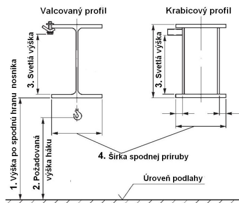
Jednonosníková mačka hlavné rozmery
